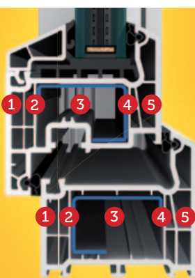
5ti komorový profil
